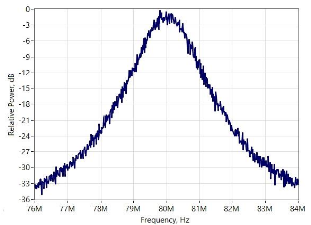
RF-line Spectrum
